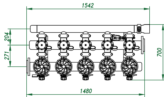
Вид сверху
