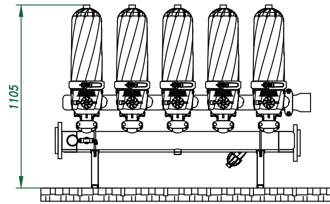
Вид спереди
