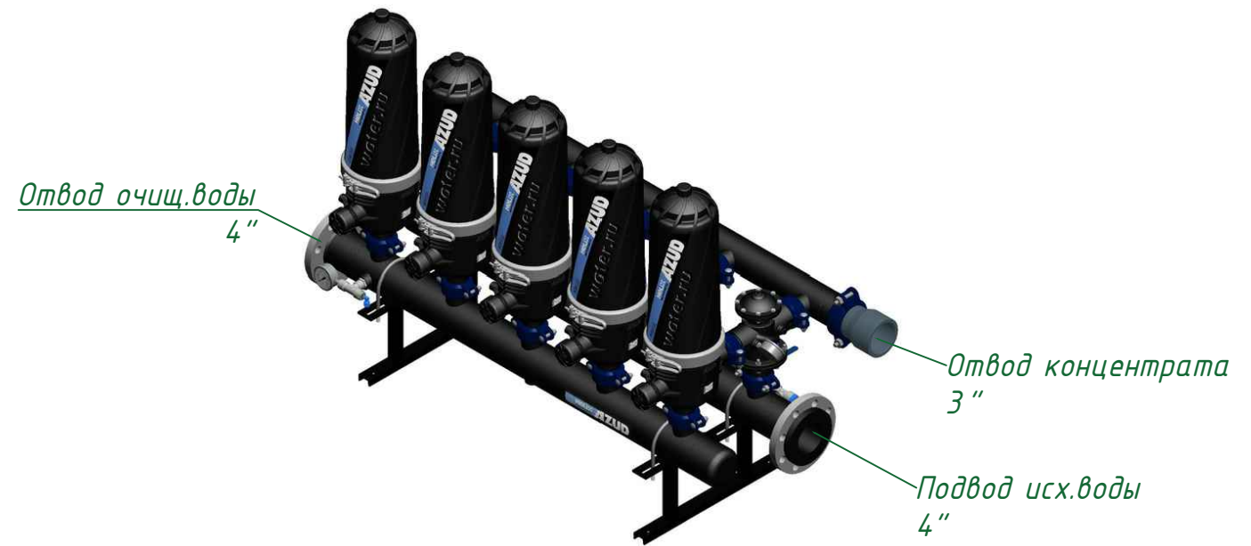
Изометрия
